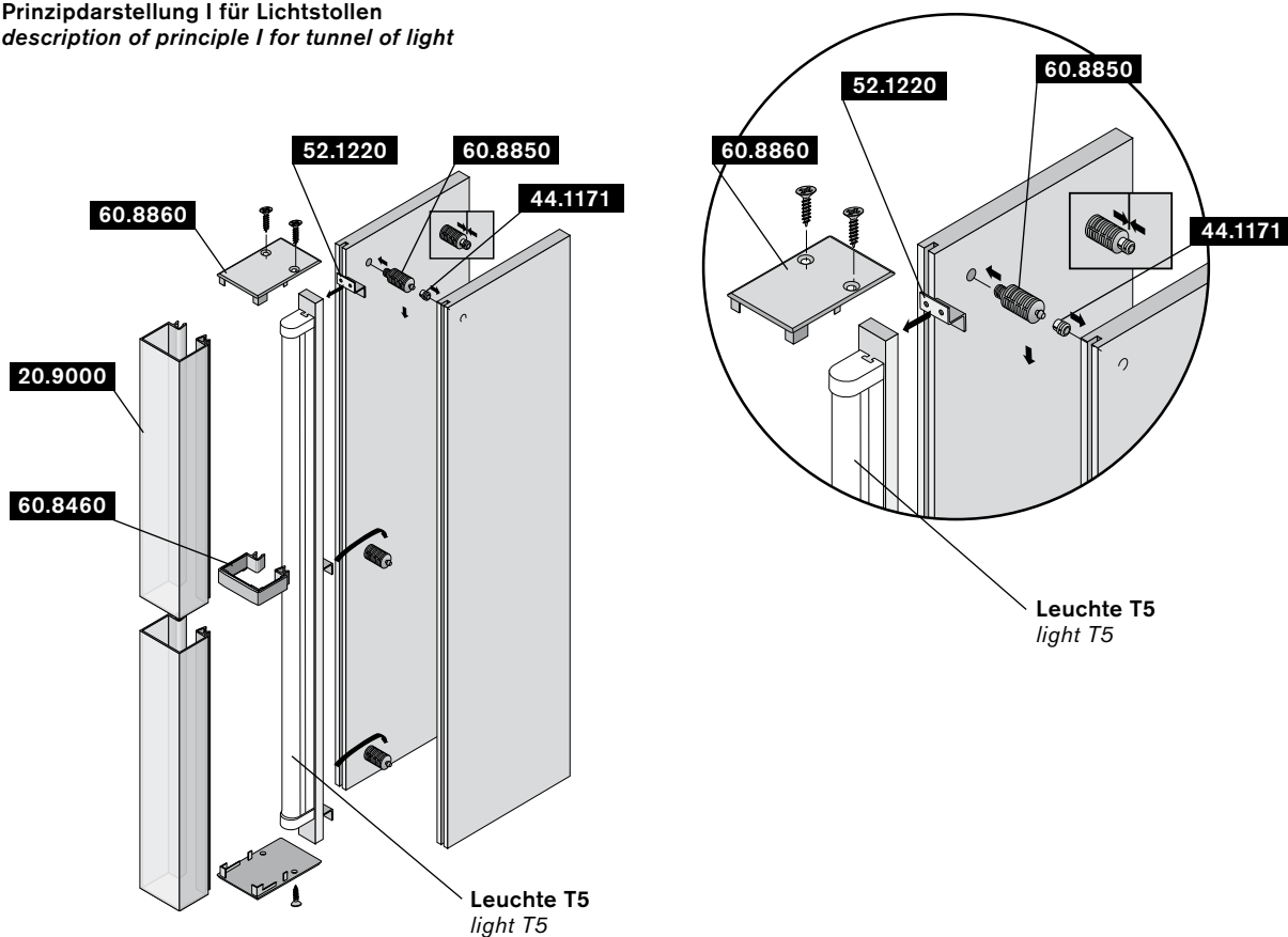
Prinzipdarstellung II für Lichtstollen description of principle II for tunnel of light
