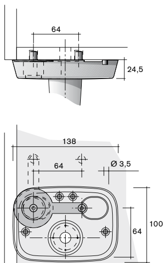
Einsatz als Eckfu mit Absttzung der Seitenwand use as corner foot for supporting carcass side
