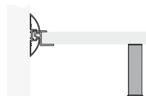
Bodenabstützung base support
