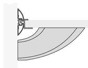
Wandabstützung wall support
